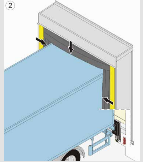
2 Körük şişirilerek bağlanan aracın etrafına sarılır ve böylece mümkün olan en iyi sızdırmazlık sağlanır.
