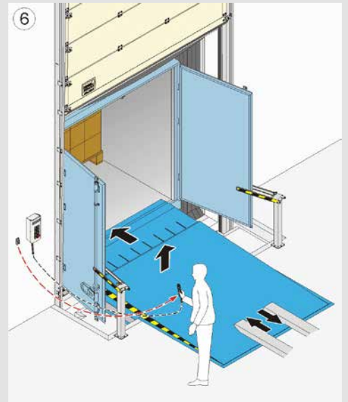
6 Yükleme rampası, araçla bağlanarak yükleme işleminin başlamasını sağlar.
