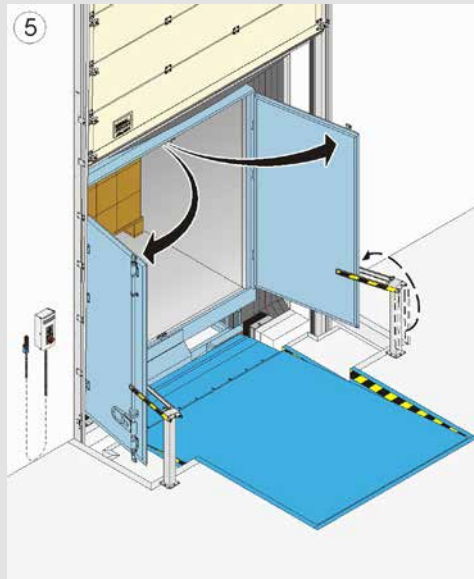
5 Kamyonun arka kapıları basamaktan açılır ve kamyon kapısı tutucularla bağlanır.
