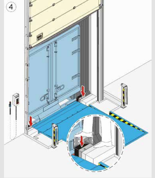
4 Yüksekliği ayarlanabilir tamponlar, aşağı indirilir ve en alçak konuma kilitlenir.
