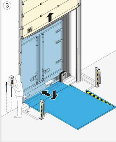
3 Seksiyonel kapı açılır ve yükleme rampasının teleskopik dudağı, araç ile bina arasındaki açıklığı kapatacak şekilde konumlandırılır.
