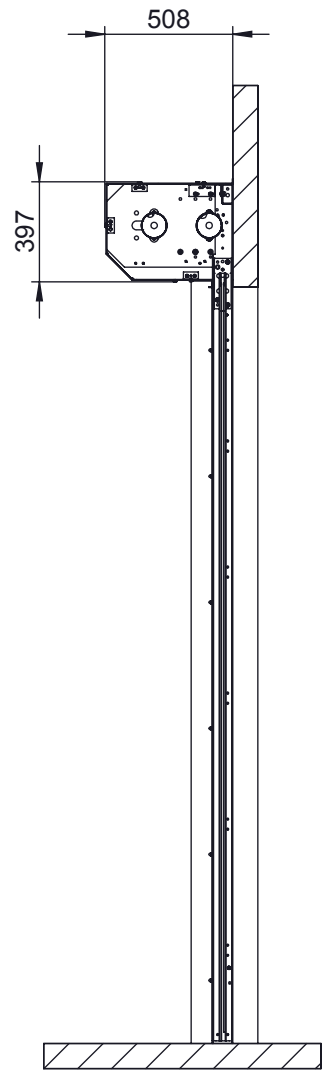
SECTION A-A
