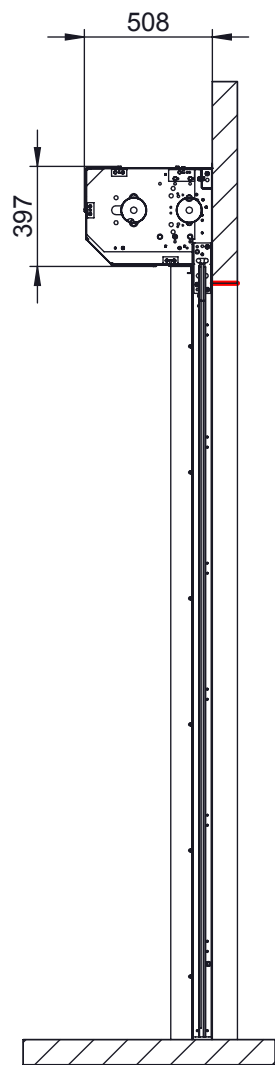
SECTION A-A
