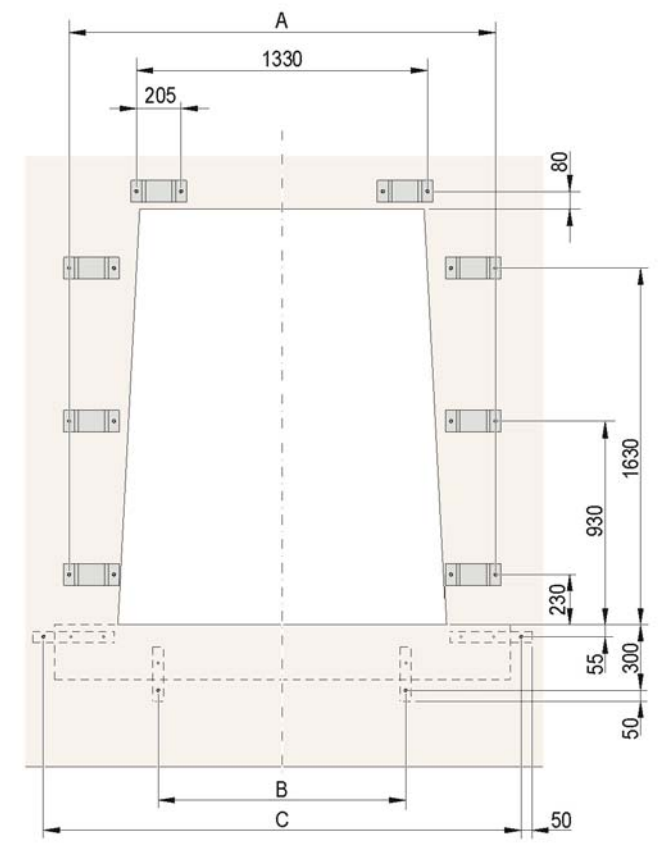
Betongvegg
