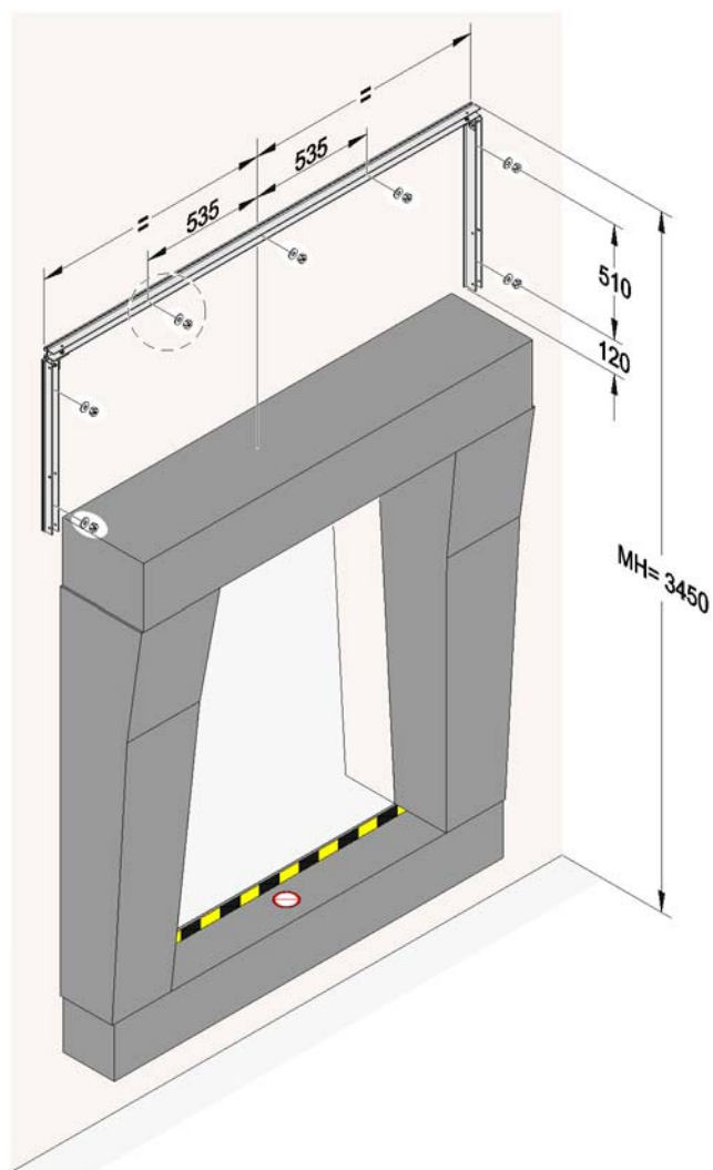
Betongvegg
