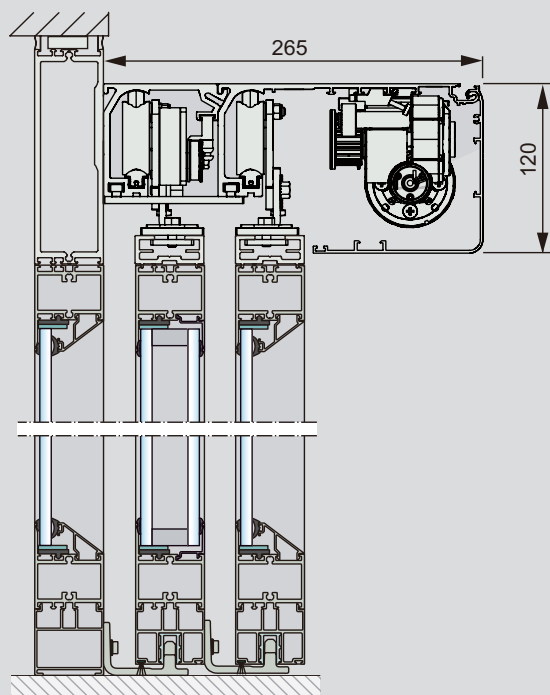
Dubbele deuren
