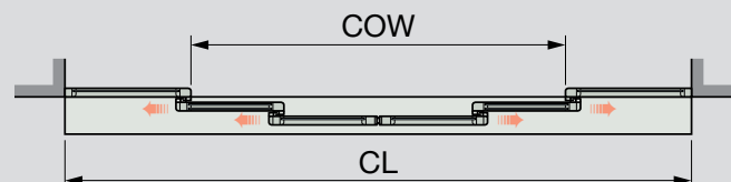
Dubbele deuren
