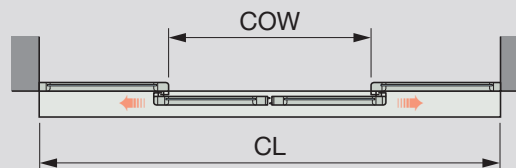
Dubbele deur
