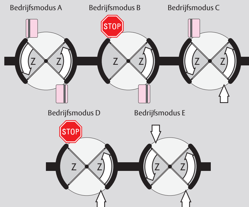
Deur met tweerichtings toegangscontrole: ASSA ABLOY RD4 A2
