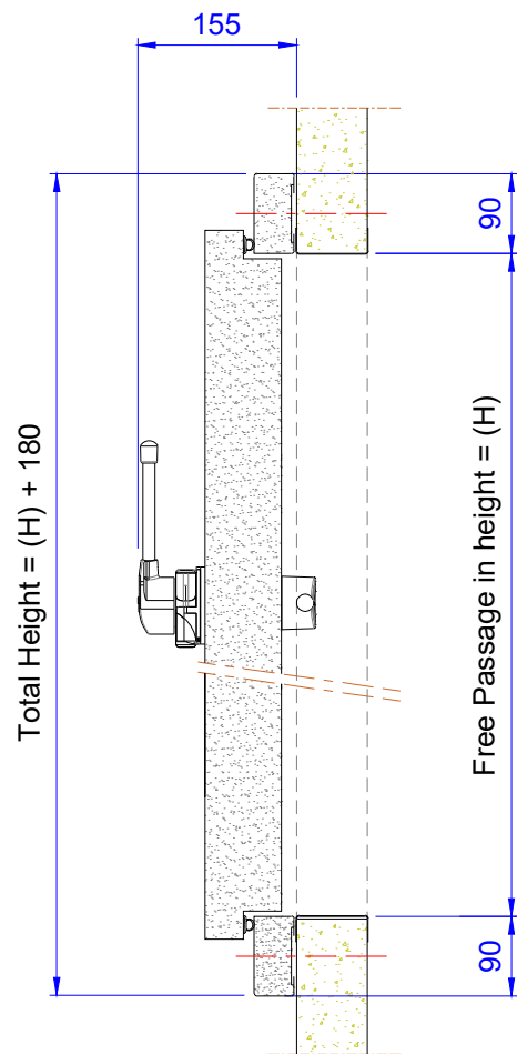
SECTION : B-B
