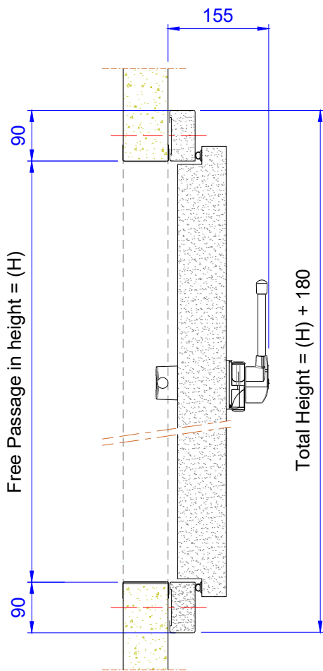
SECTION : B-B
