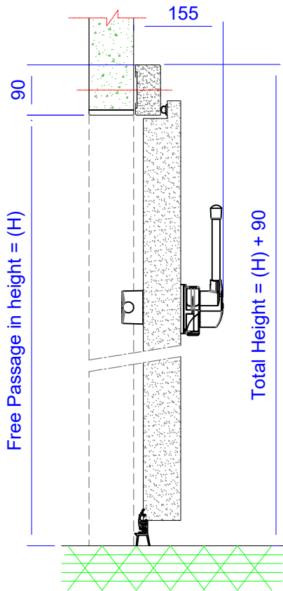
SECTION : B-B
