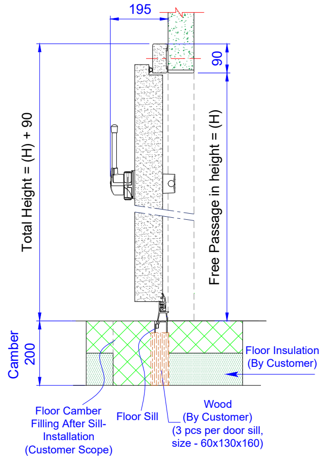
SECTION : B-B
