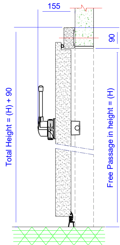
SECTION : B-B
