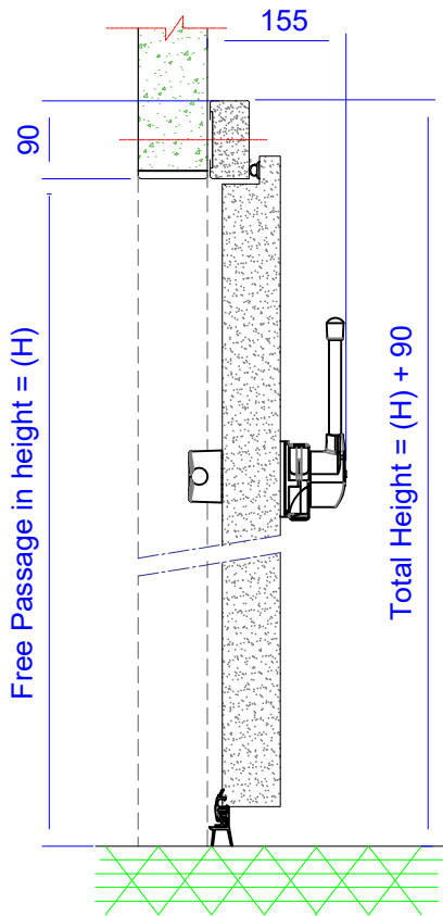
SECTION : B-B
