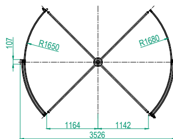
Top view, open door
