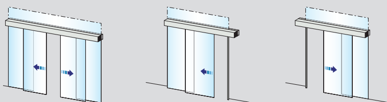
Trägermontage, Türen und Seitenteile (Oberlicht optional)
